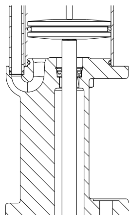
ТИП -0- Разъёмное основание, ОСНОВАНИЕ с быстроразъёмным соединением штока 65023 и ПОРШЕНЬ В СБОРЕ 67489
