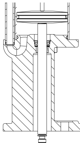
タイプ-0- 分離したベース、クイック結合ロッド 65023 ベース、67489 ピストン アセンブリ
